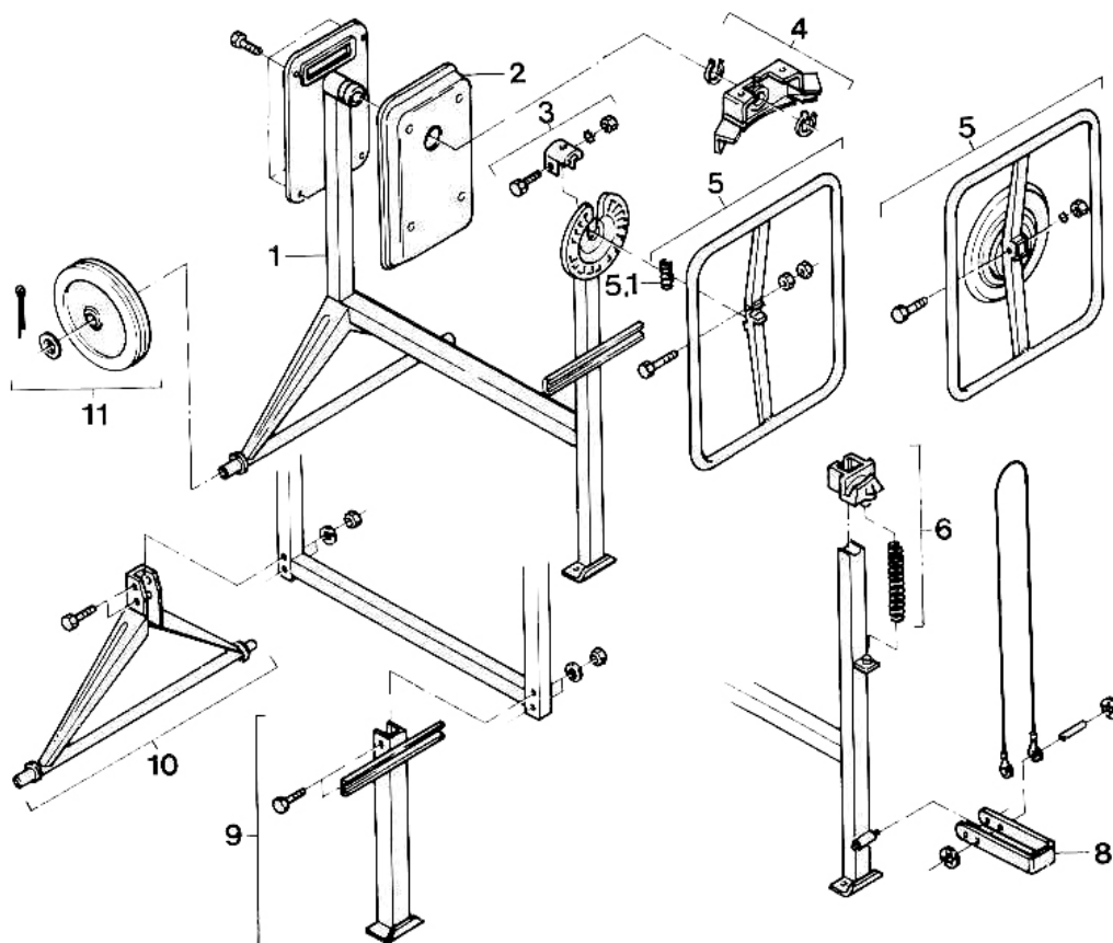
Obrázek 1, Rám míchačky
